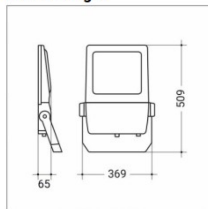
Abmessungen
