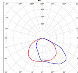
Lichtverteilung
