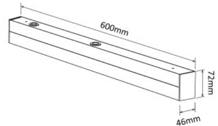
Maßskizze
