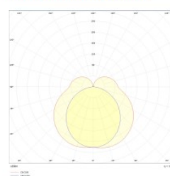
Lichtverteilungskurve
