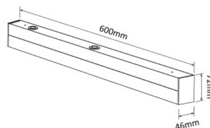
Maßskizze
